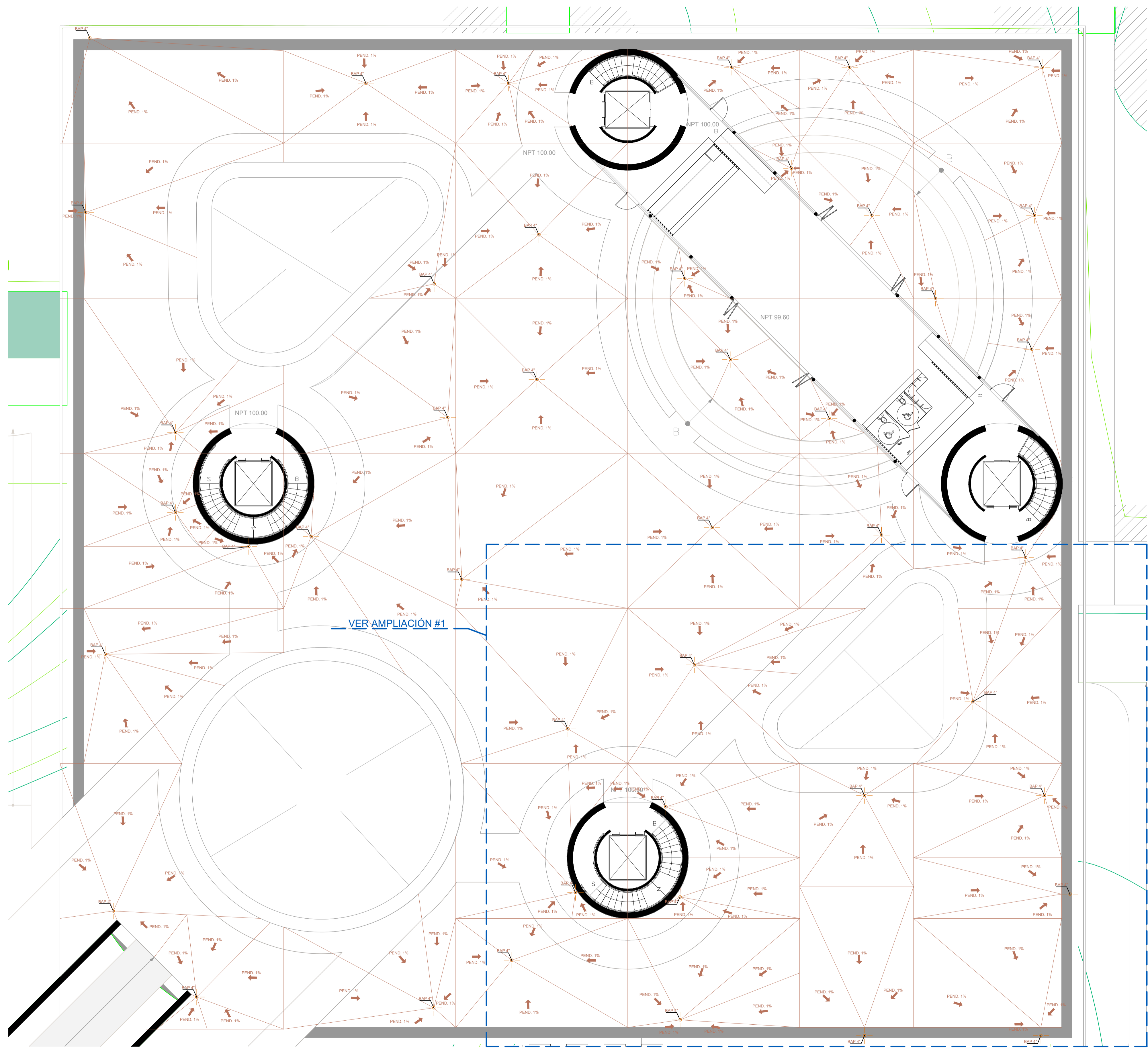
PLANO DE DRENAJES PLUVIALES TERRAZA ESCALA 1 : 150
